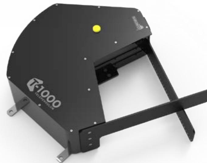
2 T-1000 telependulum
