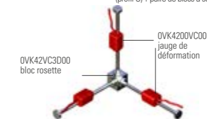
jauges de déformation en rosette 3D
