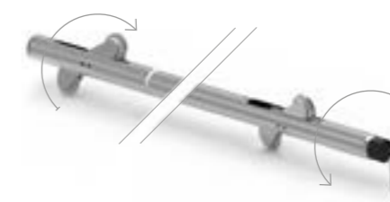
Sonde de spirauté: torsion de l'axe de la sonde pour mesurer la torsion du tube inclinométrique
