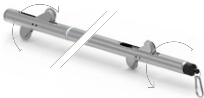
Sonda spiralometrica: torsione sull'asse della sonda per misurare la spiratura della tubazione inclinometrica
