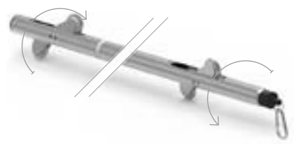
Sonda spiralometrica: torsione sull'asse della sonda per misurare la spirallatura della tubazione inclinometrica
